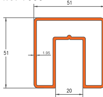
Die No. 19150 0.967 Kg/m
