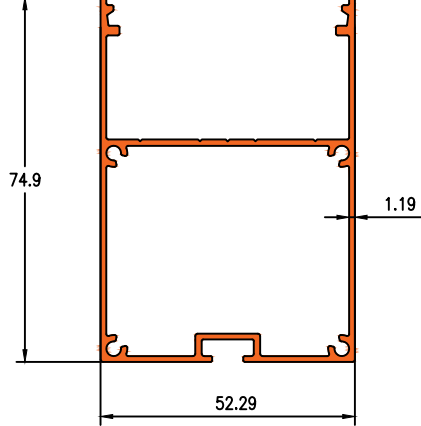
Die No. 1080 0.301KG/M
