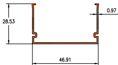
Die No. 19167 0.296KG/M
