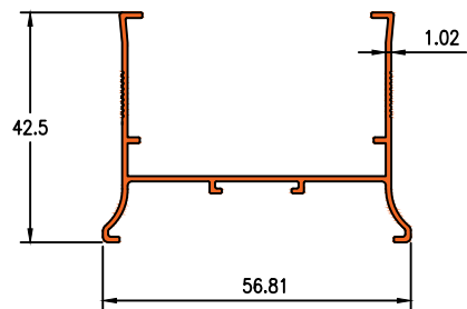
Die No. 19166 0.417KG/M
