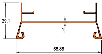
Die No. 19614 0.388KG/M
