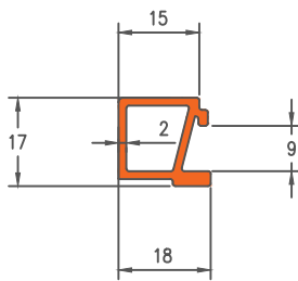
Die No. 1390 0.358Kg/m
