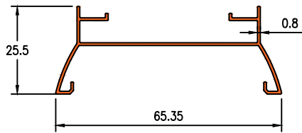
Die No. 1080 0.301KG/M
