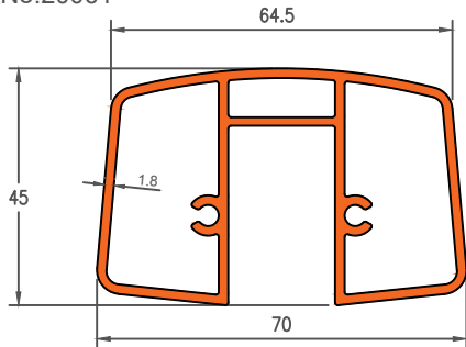
Die No. 20061 1.455 Kg/m
