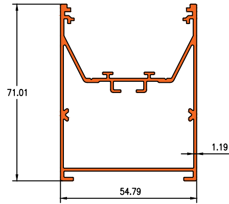
Die No. 1301 0.453KG/M
