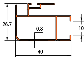
Die No. 1532 1.250 KG/12FT
