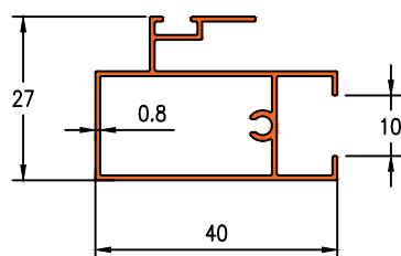
Die No. 1552 1.400 KG/12FT
