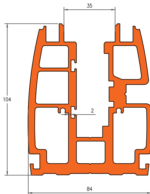
Die No. 19148 7.278Kg/m
