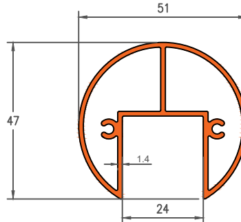
Die No. 19118 0.260Kg/m
