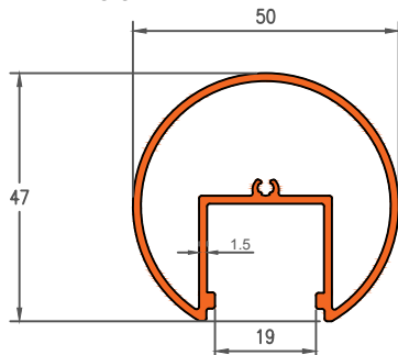
Die No. 1390 0.358Kg/m
