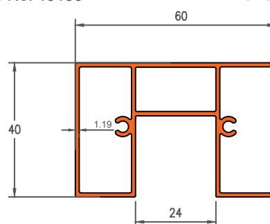
Die No. 19150 0.967 Kg/m
