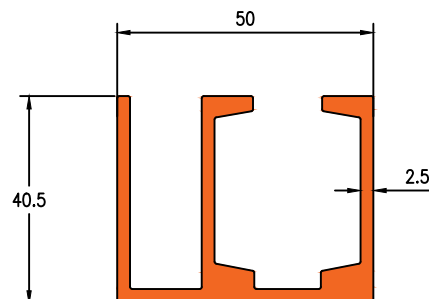
Die No. 7043 1.468Kg/m
