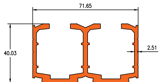
Die No. 7064 1.736Kg/m
