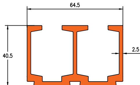
Die No. 7042 1.778Kg/m
