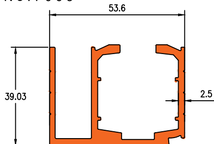
Die No. 7063 1.357Kg/m
