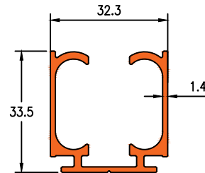
Die No. 19830 0.599Kg/m
