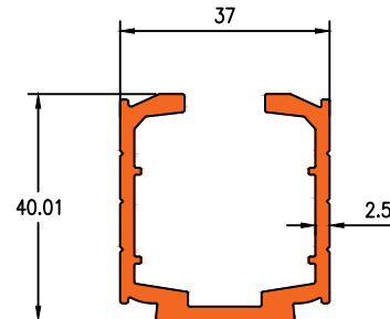
Die No. 7062 0.961Kg/m
