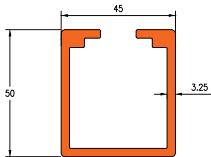
Die No. 7045 1.543Kg/m
