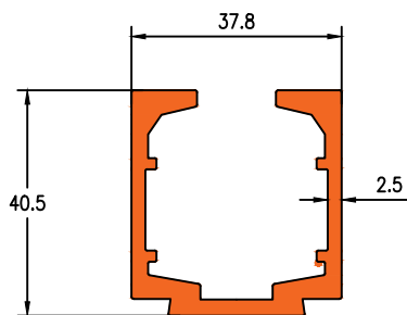
Die No. 7044 1.174Kg/m
