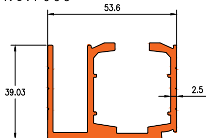
Die No. 7063 1.357Kg/m
