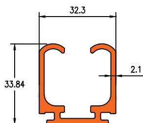
Die No. 1296 0.552Kg/m
