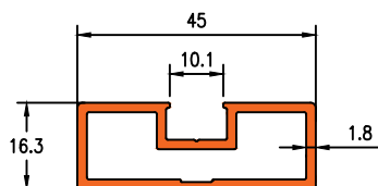
Die No. 19658 0.621Kg/m
