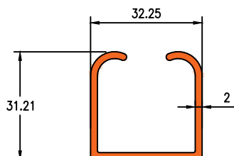
Die No. 1296 0.552Kg/m
