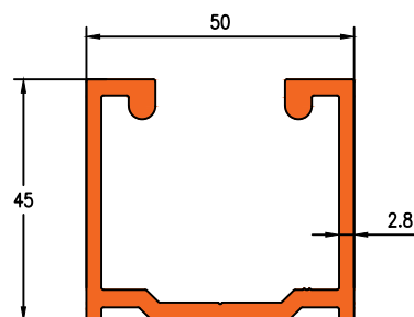
Die No. 19948 1.362Kg/m
