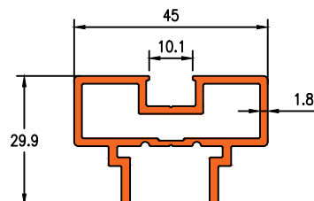
Die No. 19657 0.790Kg/m
