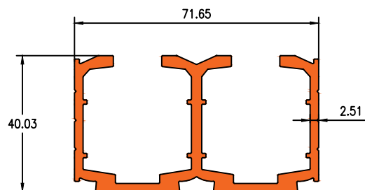
Die No. 7064 1.736Kg/m
