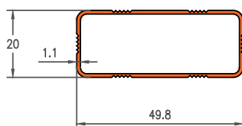
Die No. 19447
