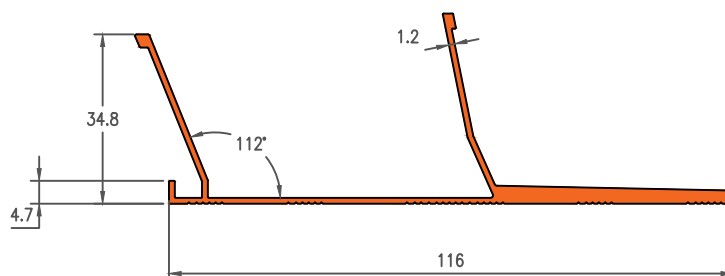
Die No. 19809
