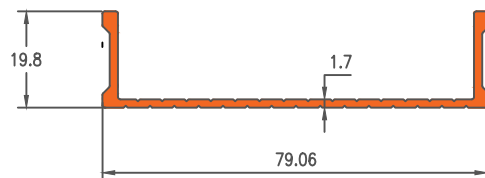
Die No. 7107
