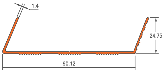
Die No. 19049
