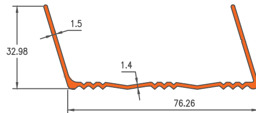
Die No. 19048
