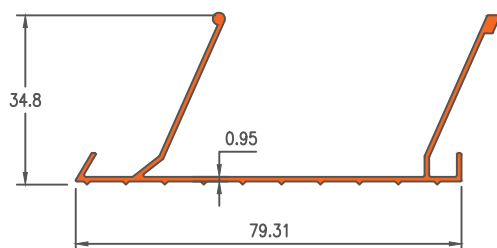
Die No. 16094
