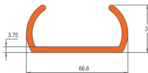
Die No. 16002
