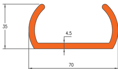
Die No. 16001
